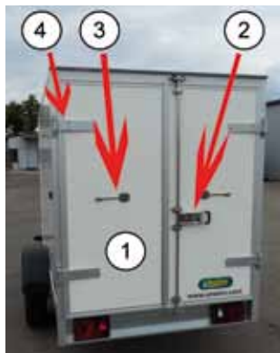
Bild: Kofferranhänger hinten
