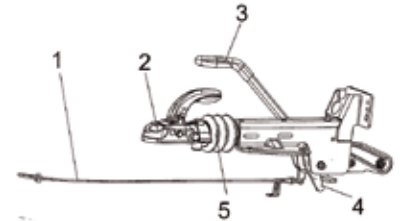
Bild 1: KNOTT Auflaufeinrichtung
