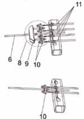
Bild 3: KNOTT Radbremse
