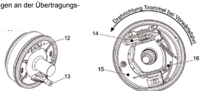
Bild 3: KNOTT Radbremse
