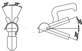
Grafik: Schwenkbereich
